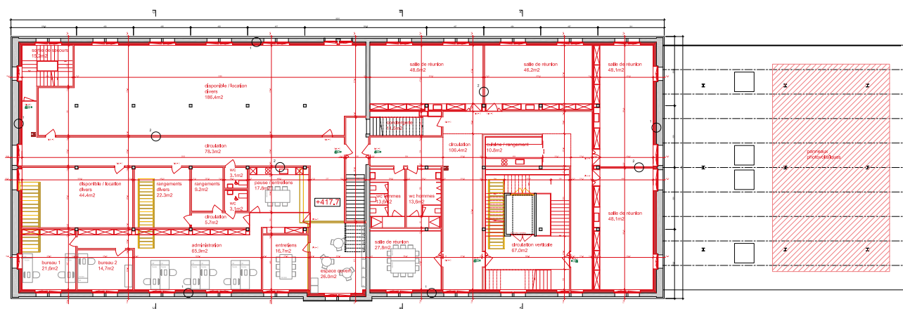
1 er étage
